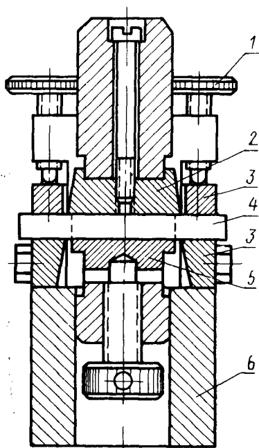
1 — винт; 2 — нож; 3 — опоры; 4 — образец; 5 — опорная плита; 6 — корпус
