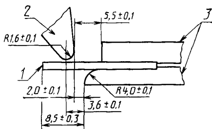
1—испытуемый образец; 2—ударная кромка; 3—зажимное устройство
