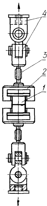
1—образец; 2—захват; 3—тяга; 4—шарнирная подвеска.
