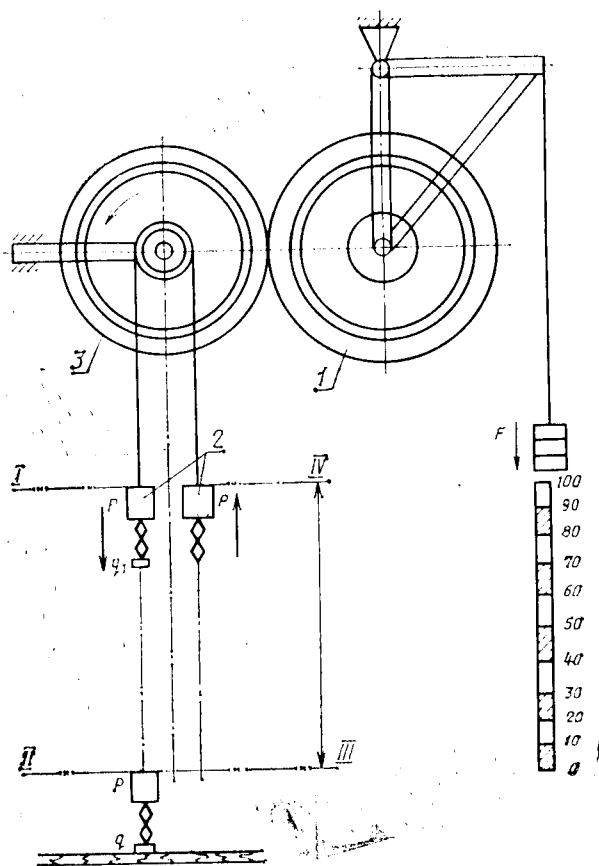
1—шина на обод; 2—грузы; 3—барабан
