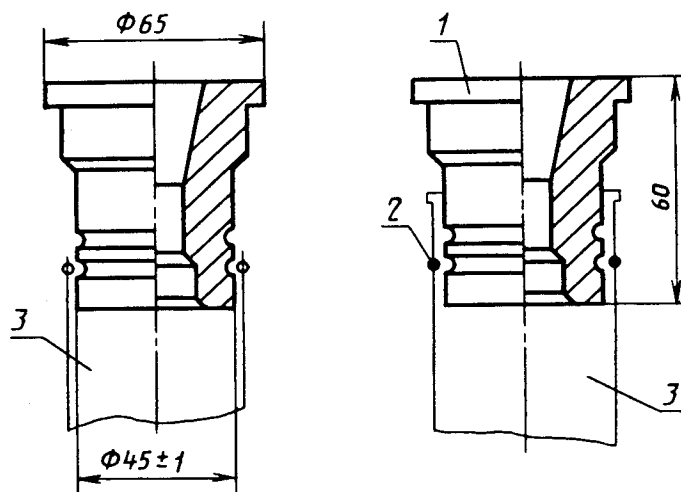
1 — патрубок; 2 — резиновое зажимное кольцо; 3 — презерватив
