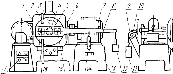
1—кожух; 2—воздуховод; 3—неравноплечий рычаг; 4—диск; 5—полый вал; 6—редуктор; 7—электромотор; 8—скоба; 9—ролик; 10—грузовой стержень; 11—постоянный груз; 12—уравновешивающий груз; 13—станина; 14—динамометр; 15—винты; 16—рамка-держатель; 17—выключатель
