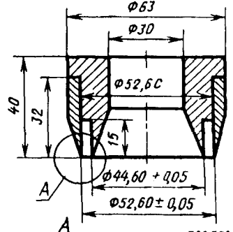
Схема ножа для вырубki кольцевых образцов
