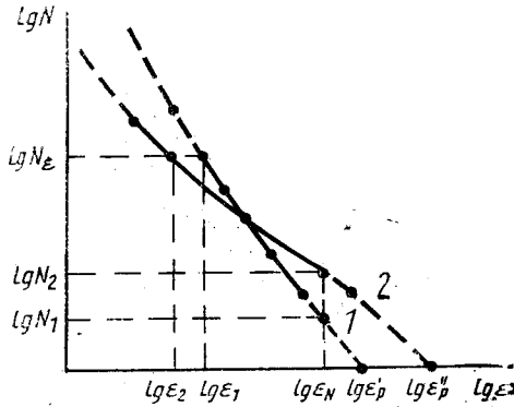
1, 2 — кривые для резин на основе различных каучуков
