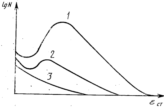
1—высокопрочные эластомеры, кристаллизующиеся при растяжении; 2—высокопрочные наполненные некристаллизующиеся резины; 3—малопрочные ненаполненные резины
