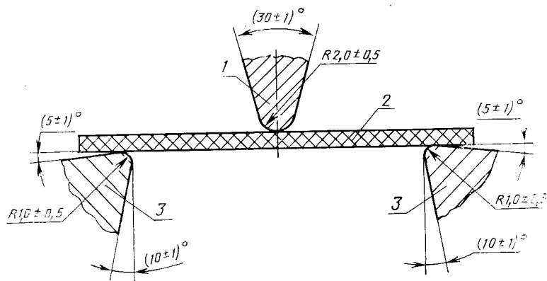
1—боек маятника; 2—образец; 3—опоры
