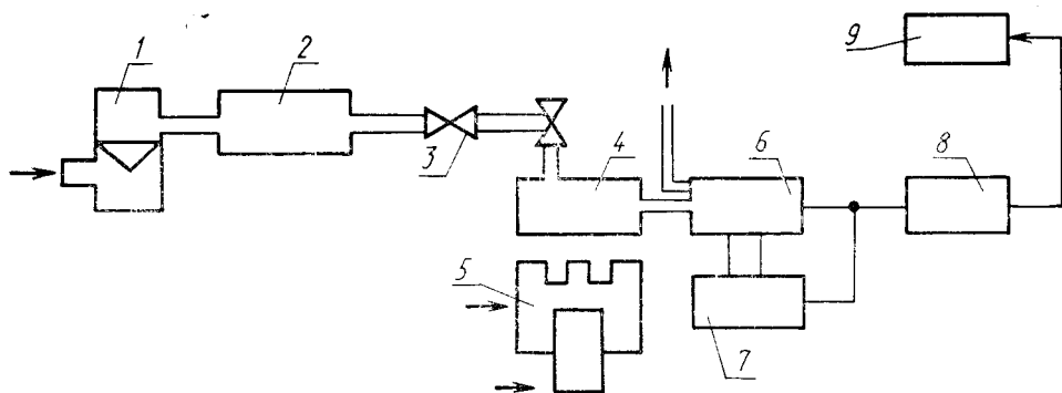
1 — расходомер газа-носителя; 2 — осушитель газа; 3 — редуктор; 4 — печь; 5 — нагреватель печи с регулятором температуры; 6 — электролитическая ячейка; 7 — источник питания электролитической ячейки; 8 — аналого-цифровой преобразователь; 9 — дисплей
