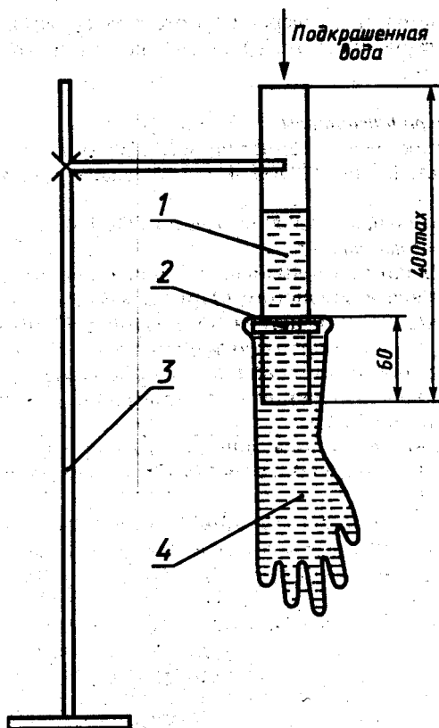
1 — цилиндр; 2 — муфта; 3 — опорная стойка; 4 — испытываемая перчатка
