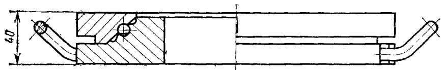
Исполнение 2
