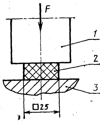
1 — силовой цилиндр (плунжер); 2 — образец типа 1; 3 — нагревательная плита
