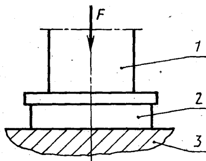
1 — плунжер; 2 — образец типа 3; 3 — нагревательная плита
