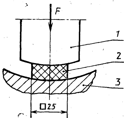
1 — силовой цилиндр (плунжер); 2 — образец типа 2; 3 — нагревательная плита
