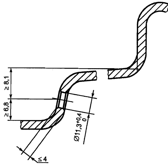
Рисунок 3 — Размеры вентиляного отверстия для бескамерных шин
