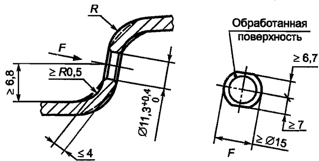
Рисунок 4 — Исполнение поверхности в зоне вентиляного отверстия
