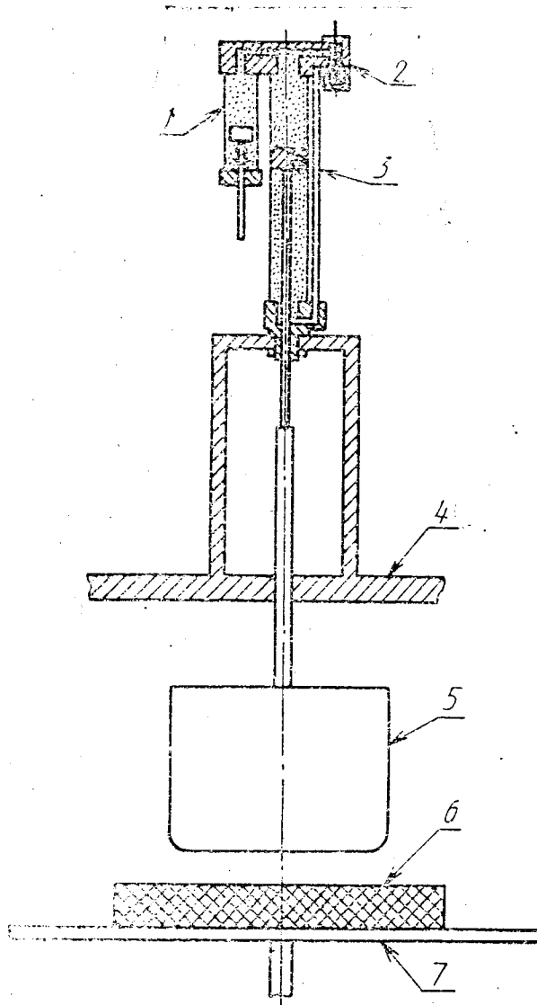
Схема устройства с автоматическим регулированием индентора
