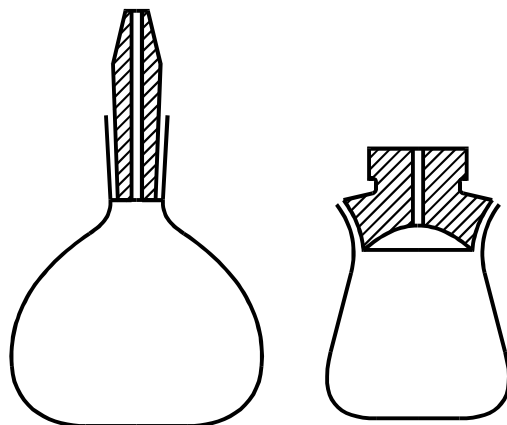
Рисунок 1 — Пикнометры
