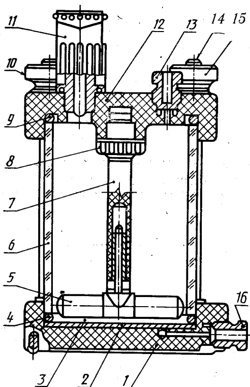
Схема ячейки для испытания мембран
