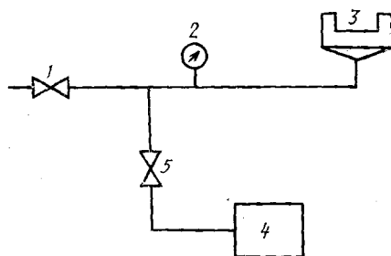
Установка для определения точки пузырька мембран
