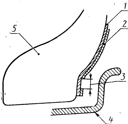
Давление посадки на обод — электрический метод
