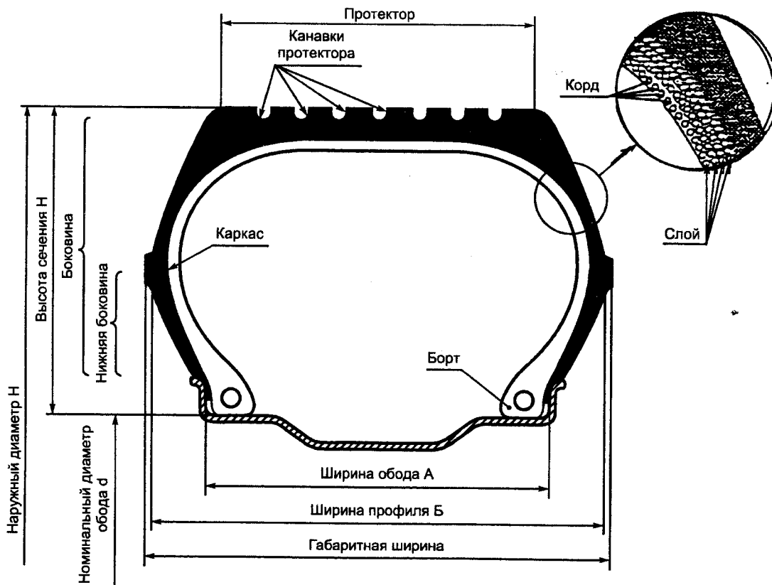
Рисунок 1 — Конструкция пневматической шины (см. раздел 2 Правил)
