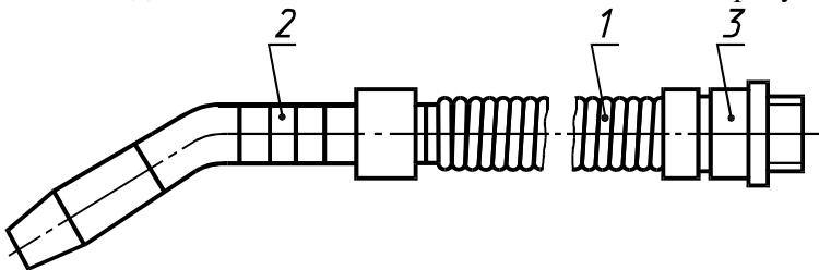
1 — рукав; 2 — наконечник; 3 — патрубок
