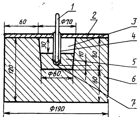
1—термопара, соединенная с самописцем; 2—крышка; 3—реакционный сосуд (картонный стакан); 4—пробирка; 5—реакционная смесь (смола); 6—пеноблок; 7—гликоль
