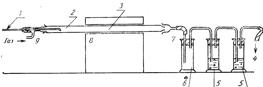
Агрегат трубчатой печи
