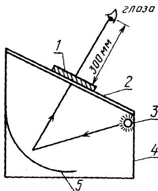
1—испытуемая пластинка; 2—стекло; 3—источник света; 4—коробка; 5—пластина алюминиевая
