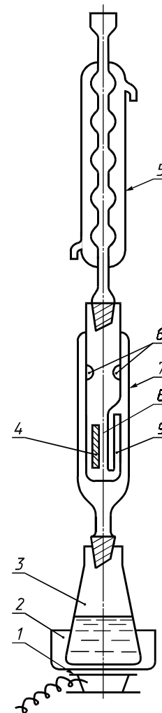
1 — электроплитка; 2 — песочная баня; 3 — колба с n -гептаном; 4 — патрон с полимером; 5 — шариковый холодильник; 6 — отверстия; 7 — экстрактор; 8 — ловушка экстрактора; 9 — сифон
