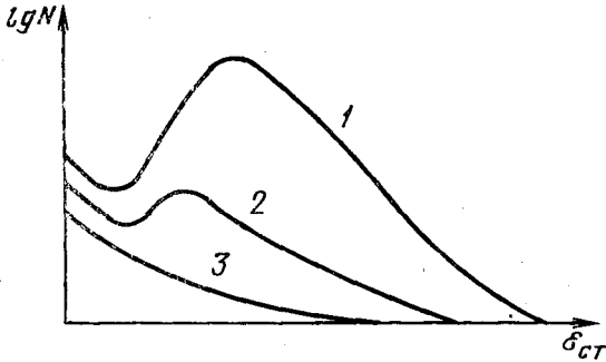
1—высокопрочные эластомеры, кристаллизующиеся при растяжении; 2—высокопрочные наполненные некристаллизующиеся резины, например, из бутадиен-стирольного каучука; 3—малопрочные неаполненные резины
