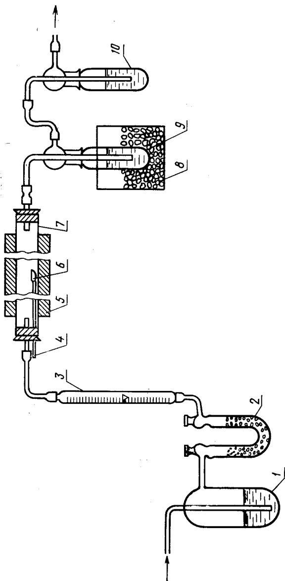
1—промывная склянка, наполненная поглотительным раствором; 2—У-образная сушильная трубка, наполненная безводным хлоридом кальция; 3—расходомер; 4—термометр или термометр из кварцевого стекла; 5—трубчатая печь; 6—лоточка для прокаливания; 7—кварцевая или стальная трубка; 8—сосуд Дьюара, наполненный твердой двуокисью углерода; 9, 10—промывная склянка, наполненная трихлорэтиленом
