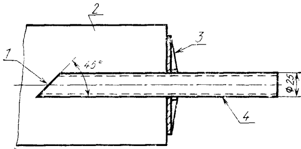
1—центр мешка; 2—мешок; 3—горловина мешка; 4—трубка
