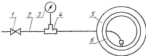
1—вентиль; 2—трубопровод; 3—манометр; 4—тройник; 5—шина; 6—обод
