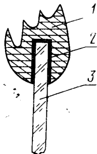
1—резиновый уплотнитель; 2—мастика; 3—стекло
