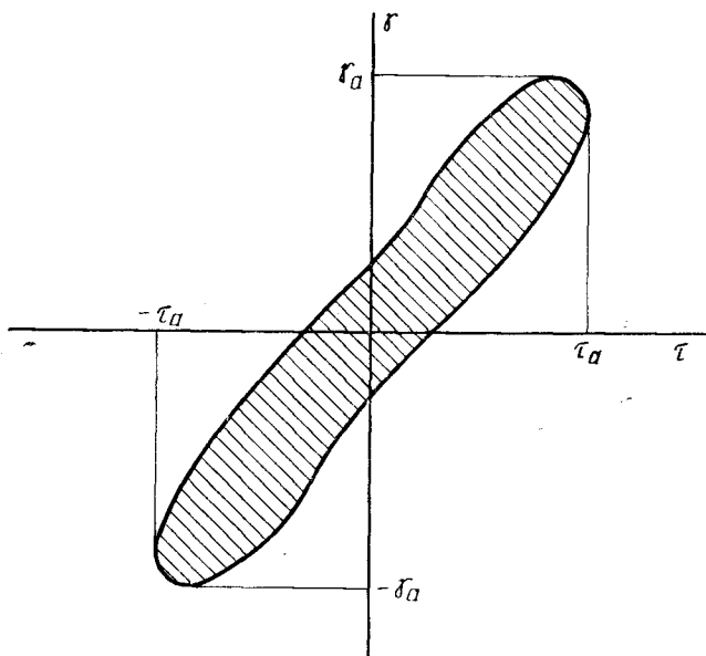
\delta_a — амплитуда деформации; \tau_a — амплитуда напряжения
