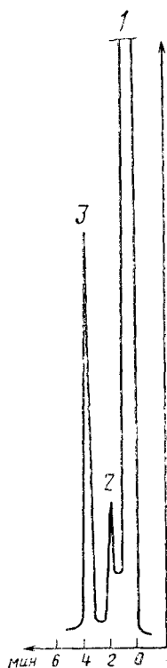
Хроматограмма свободного стирола
