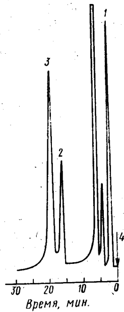
Хроматограмма фенолоформальдегидных смол, содержащих ацетон
