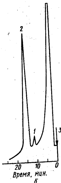
Хроматограмма фенолоформальдегидных смол
