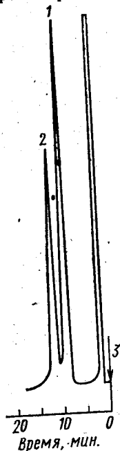
Хроматограмма фенолоформальдегидных смол
