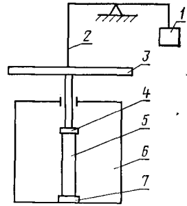
1—противовес; 2—провода; 3—инерционная деталь; 4—верхний подвижный зажим; 5—образец; 6—термостатирующая камера; 7—нижний неподвижный зажим
