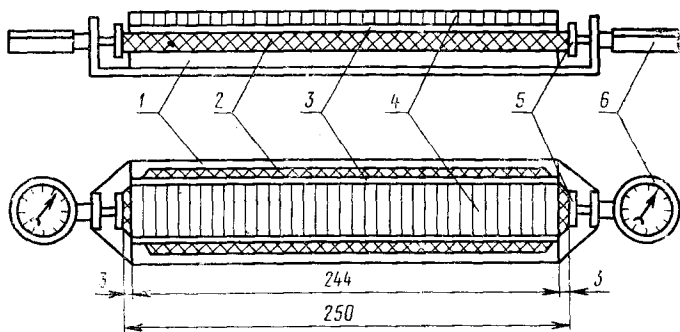
1—стальная плита; 2—испытуемый образец; 3—металлический вкладыш длиной 244 мм; 4—прижимной груз; 5—головка индикатора с металлическим диском диаметром 16 мм и толщиной 1 мм; 6—индикатор с точностью измерения 0,01 мм
